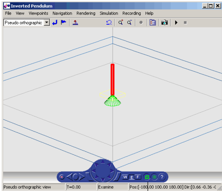
Wireframe toggle
